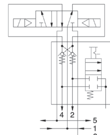
Модуль промежуточной позиции (5/2)
