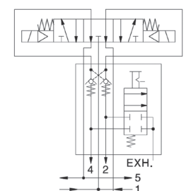
Модуль промежуточной позиции (5/3)
